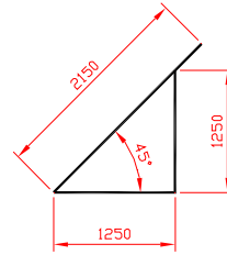
Dimensiones de los perfiles del triángulo soporte
